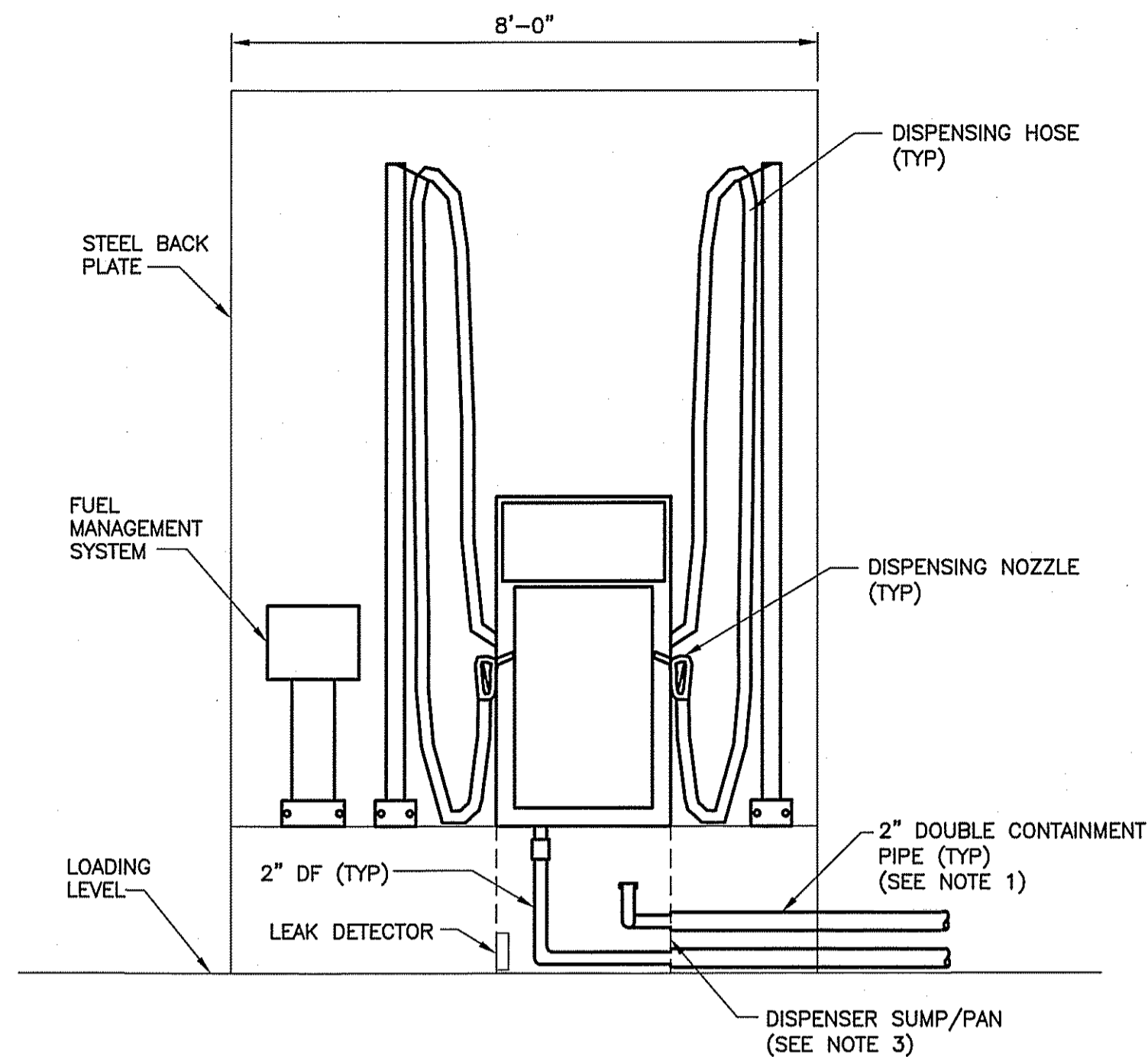
SECTION A SCALE: 1/2"=1'-0"
