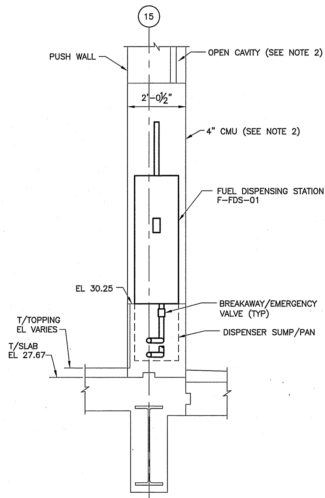
SECTION B SCALE: 1/2"=1'-0"
